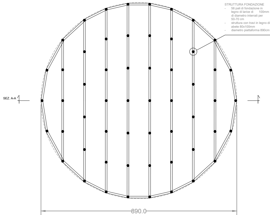
PIANTA STRUTTURA PAVIMENTO
