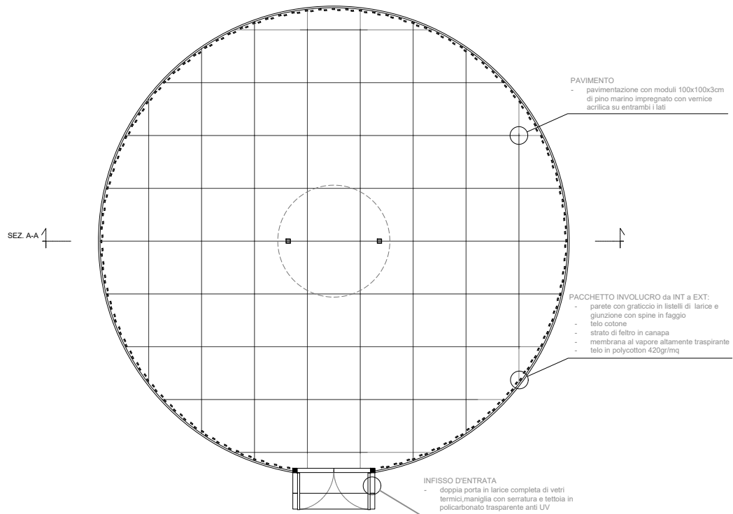
PIANTA STRUTTURA PAVIMENTO
