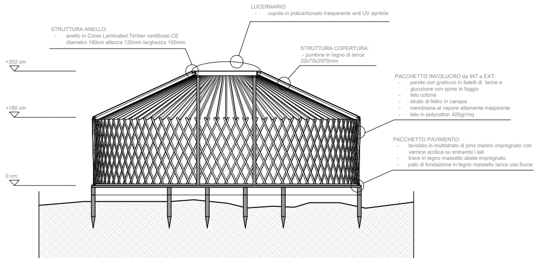
SEZIONE A-A - ARCHITETTURA
