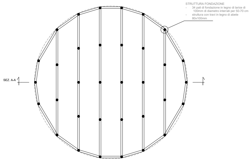
PIANTA STRUTTURA PAVIMENTO
