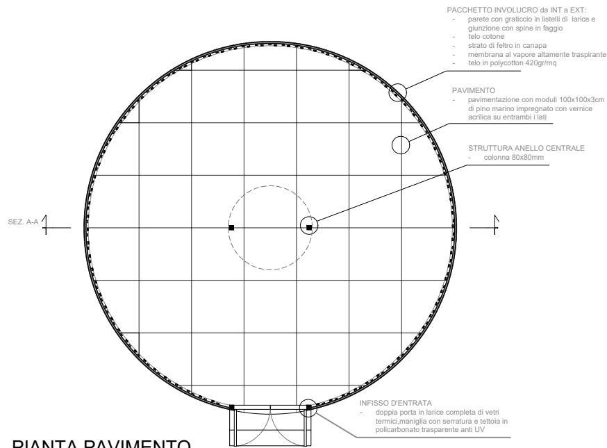
PIANTA PAVIMENTO
